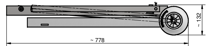
Untergestell zusammengeklappt Frontbleche im Bodenblech verstaут
