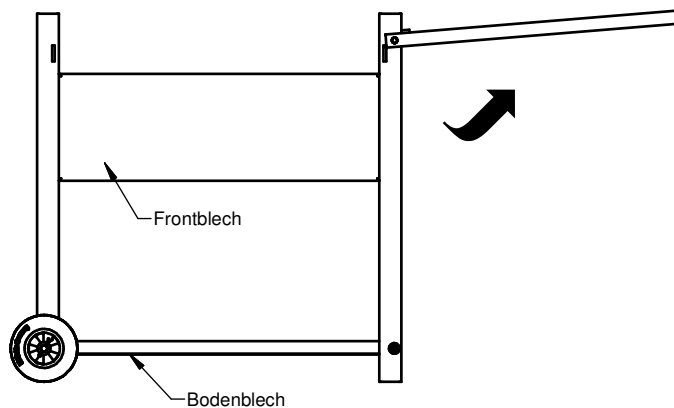
Untergestell mit hochgeklappten Griffen
