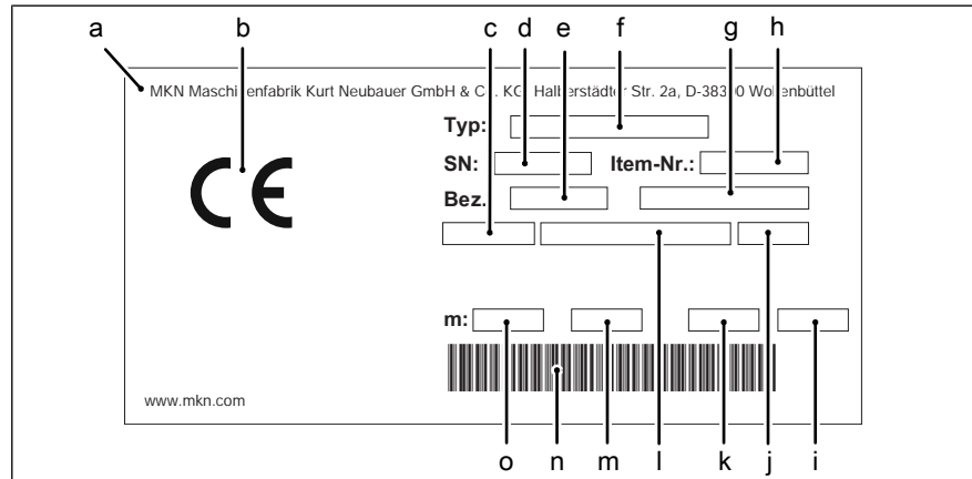
Bild: Typenschild-Angaben
